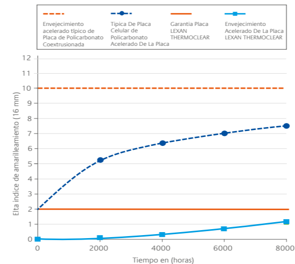
Figura 1: Índice de amarilleamiento llevado a cabo con ATLAS CI5000 (ISO 11341 / ASTM G155).
