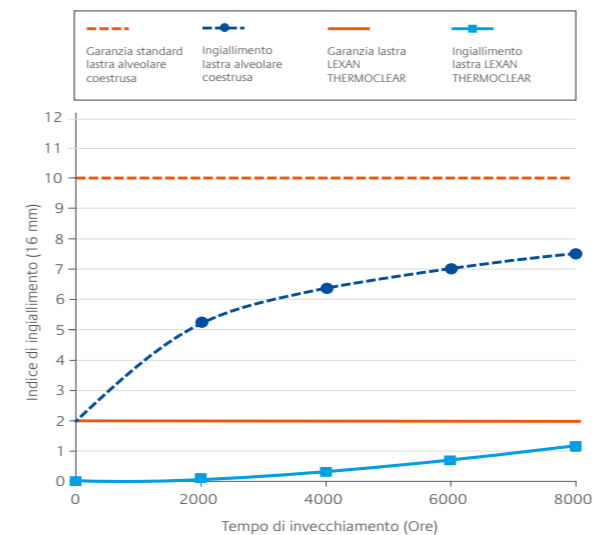
Figure 1: Tabella dell'Indice di ingiallimento ATLAS Ci500 (ISO 11341 / ASTM G155)
