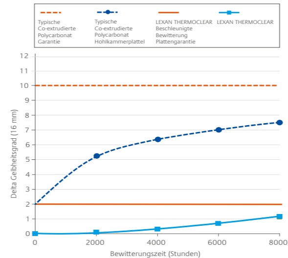
Zeichnung 1: Gelbheitsgrad Index durch ATLAS Ci5000 (ISO 11341 /ASTM G155) Witterung
