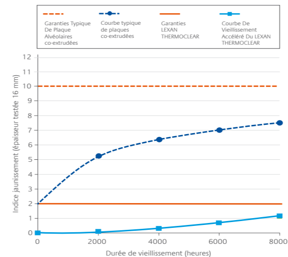
Figure 1: Indice de jaunissement en fonction du temps ATLAS CI500 (ISO 11341 / ASTM G155)
